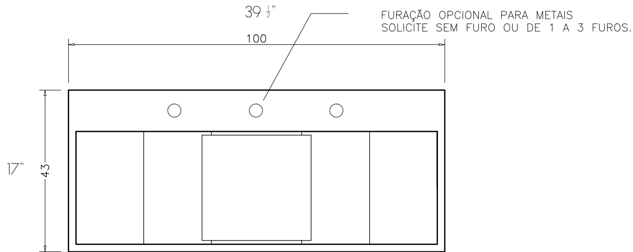
SUPERIOR / TOP
